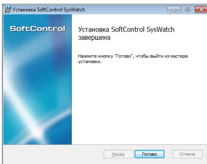
Рисунок 7. Завершение установки
