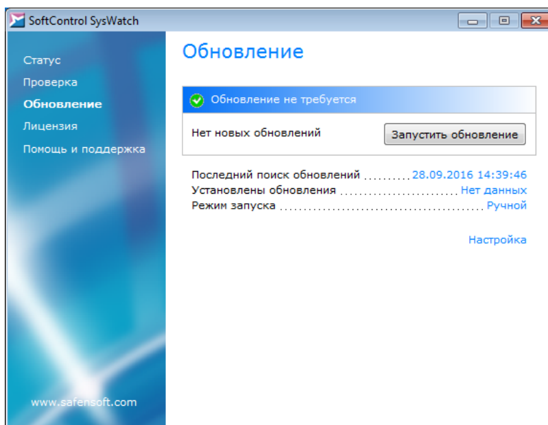
Рисунок 30. Вкладка "Обновление"
