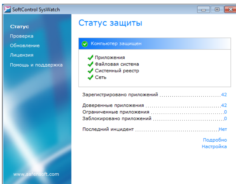
Рисунок 28. Вкладка "Статус"
