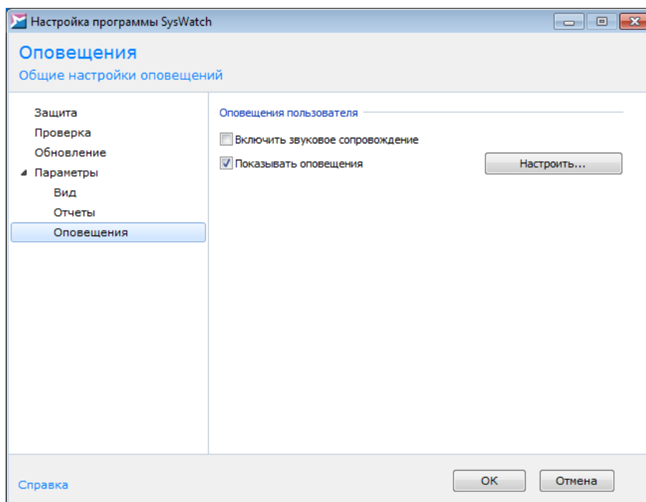
Рисунок 34. Настройка оповещений
