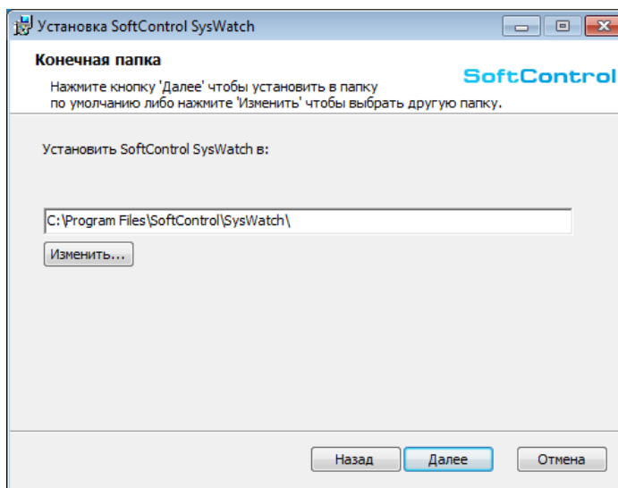
Рисунок 3. Путь установки
