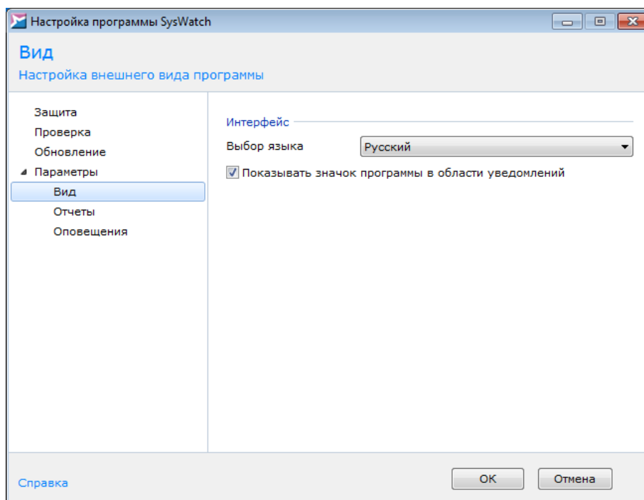
Рисунок 33. Настройка интерфейса
