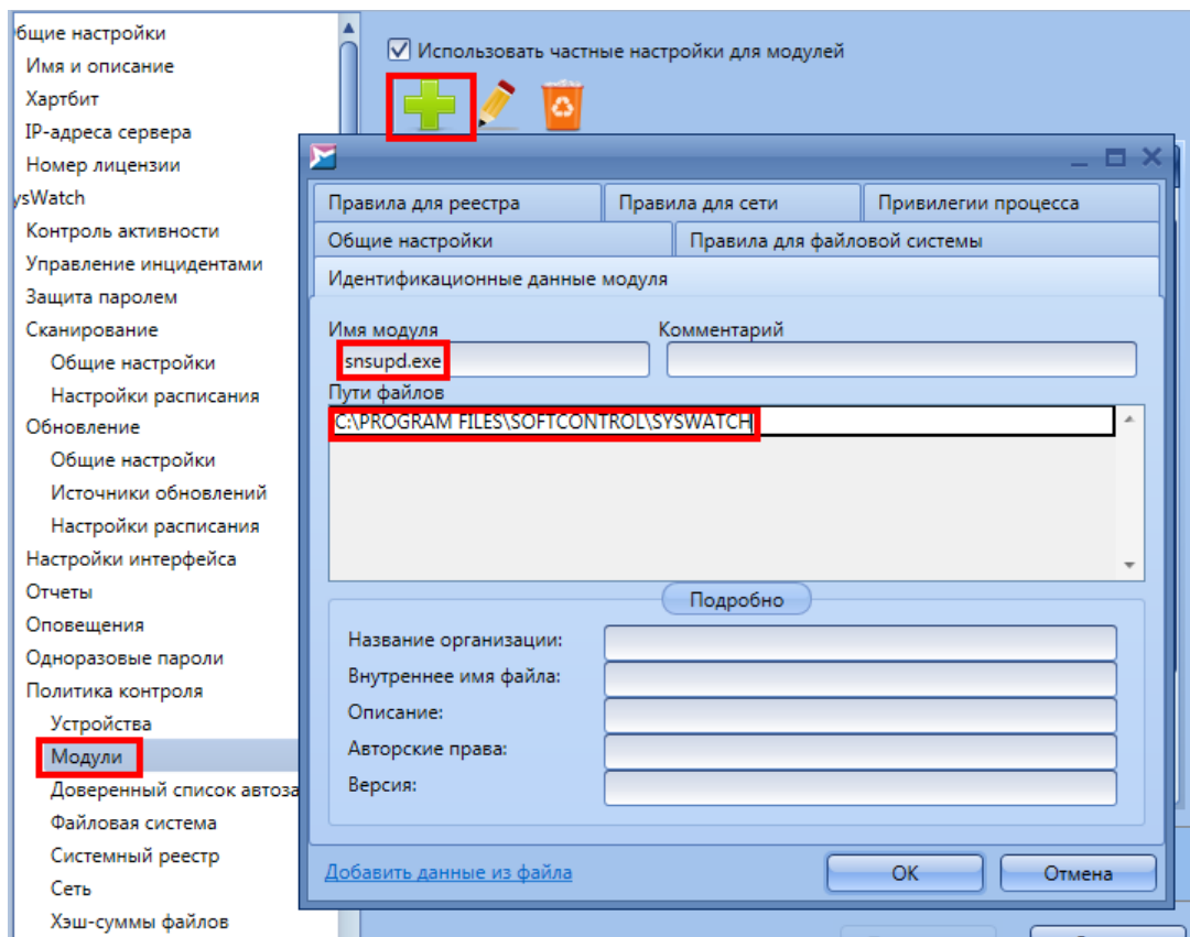
Рисунок 1. Настройка модуля обновления на примере SoftControl SysWatch
