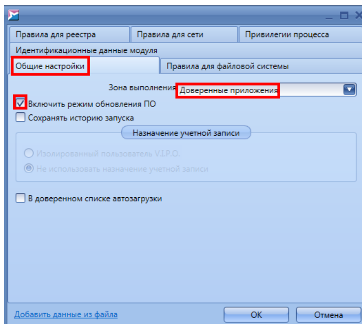
Рисунок 2. Добавление модуля в доверенные приложения
