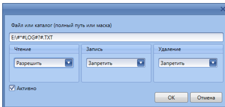
Рисунок 70. Создание правила для объекта файловой системы
